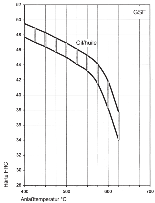
Anlaßschaubild 60ø, 930°C Öl
